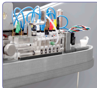
Дополнительный ионоселективный блок (ИСБ) для измерения ионов натрия, калия и хлора.
